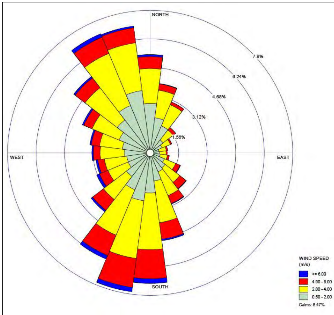
Figure 3-1 – Rose des vents pour l'aéroport de Maniwaki
