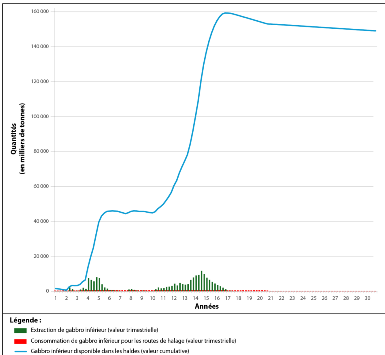
Figure R-2-40 Disponibilité du gabbro inférieur pour la surface de roulement des routes de halage
