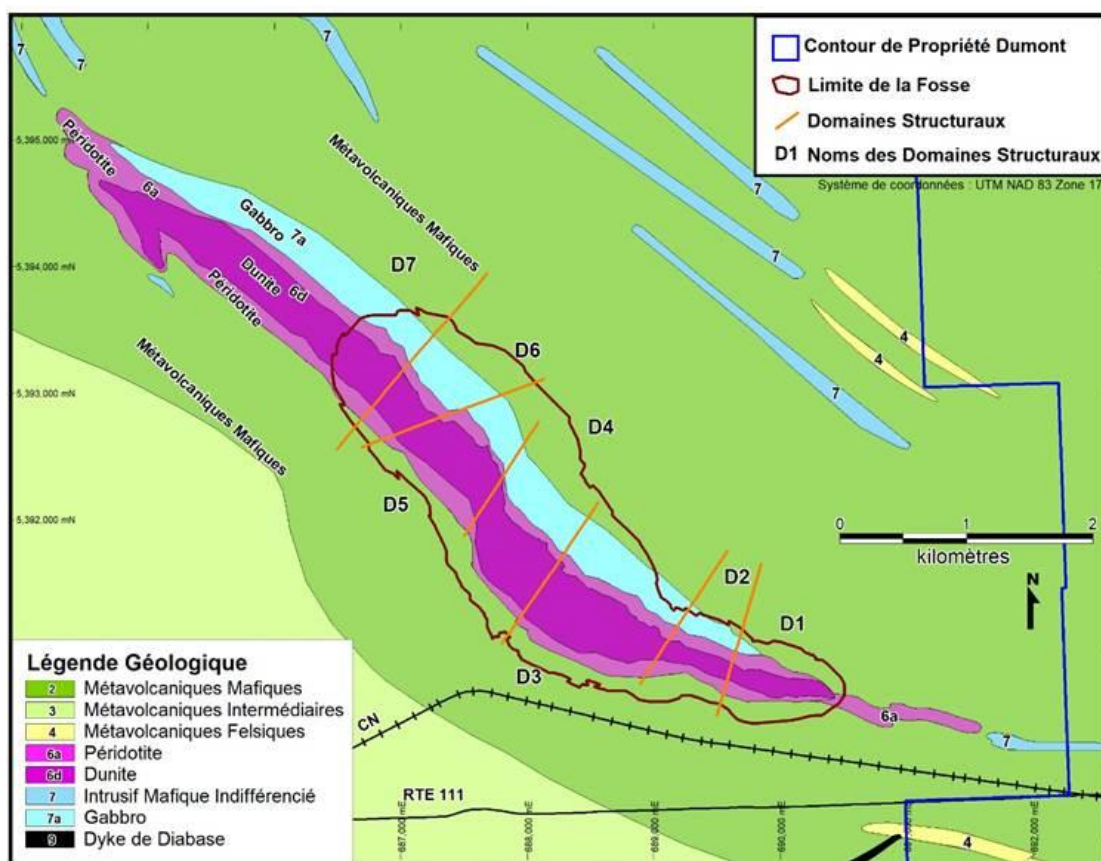
Figure R-2-38-2 Carte géologique du projet Dumont montrant les lithologies présentes au niveau du gisement
