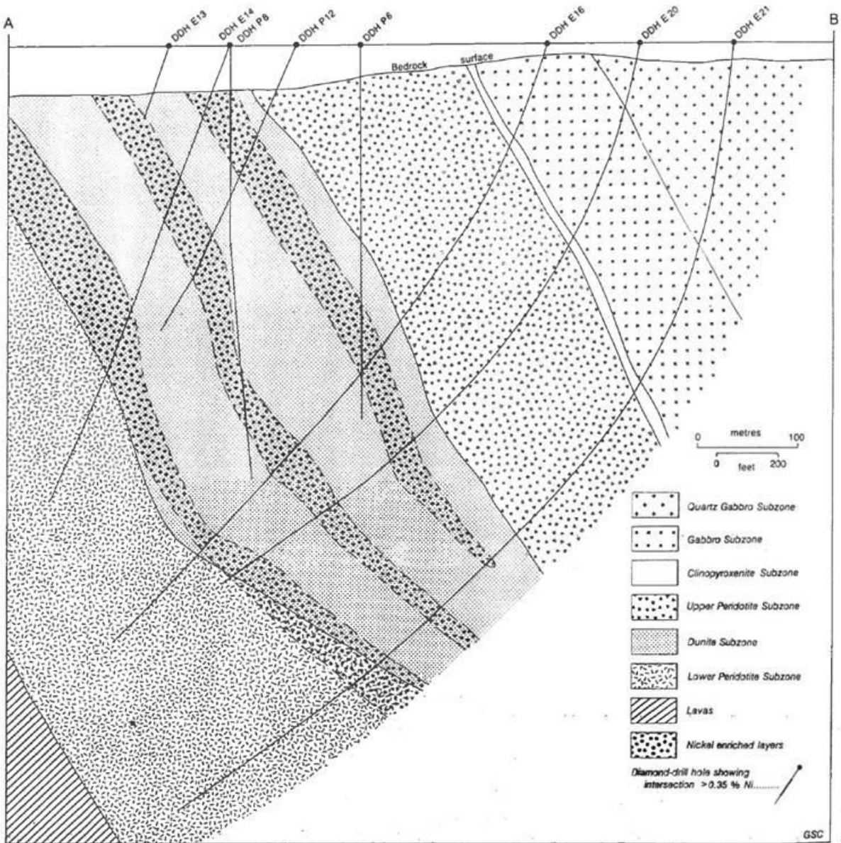
Figure R-2-38-3 Section 36+00 ouest à travers l'intrusion Dumont
