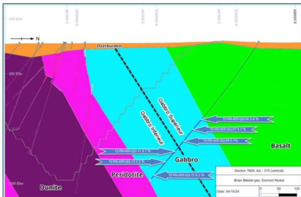
Figure R-2-38-1 Section montrant les différentes lithologies présentes dans la fosse et les teneurs en silice dans le gabbro supérieur et le gabbro inférieur
