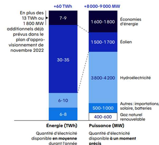
Ajouts d'énergie et de puissance d'ici 2035
