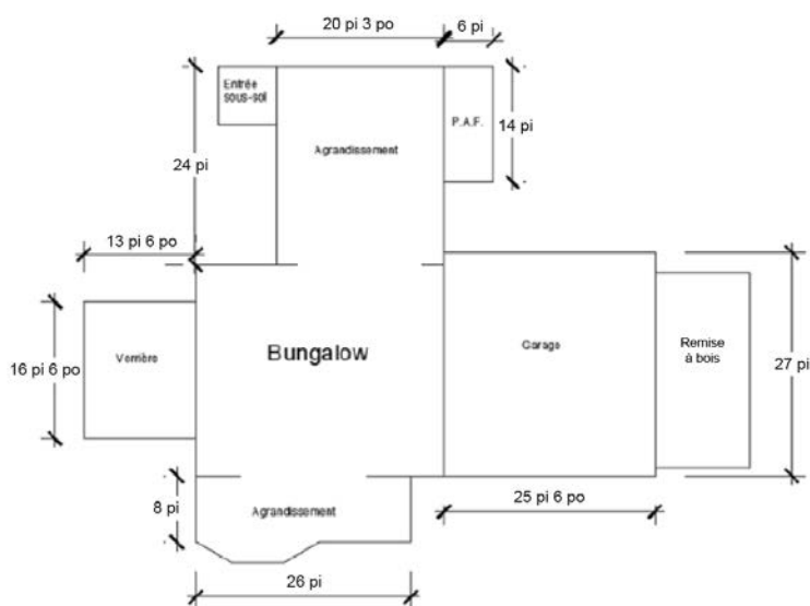
Figure 4 : Plan schématique du bâtiment situé sur la propriété
