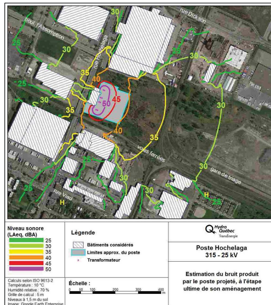
Figure 5-1 : Résultats de l'estimation du bruit continu du poste
