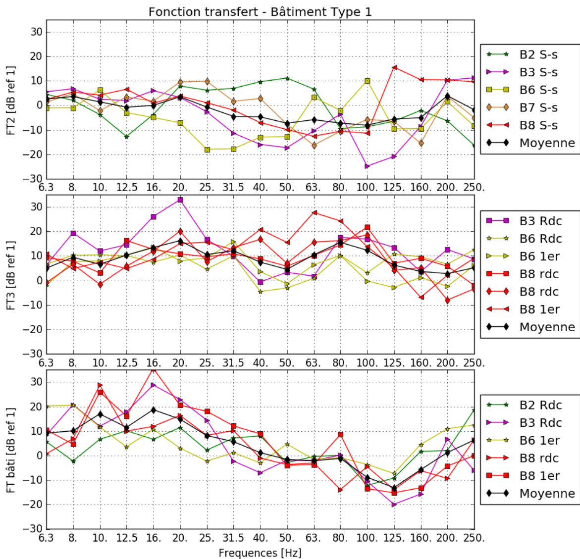
Figure 28 : Fonctions de transfert sol/bâtiment (FT2, FT3 et FTb) mesurées pour plusieurs bâtiments de type 1
