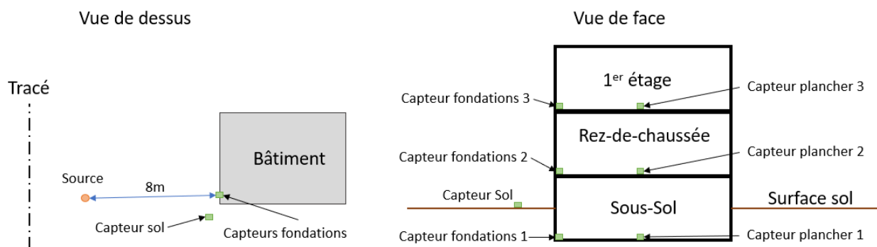
Figure 27 : Configuration des essais de mesure des fonctions de transfert sol/bâtiment
