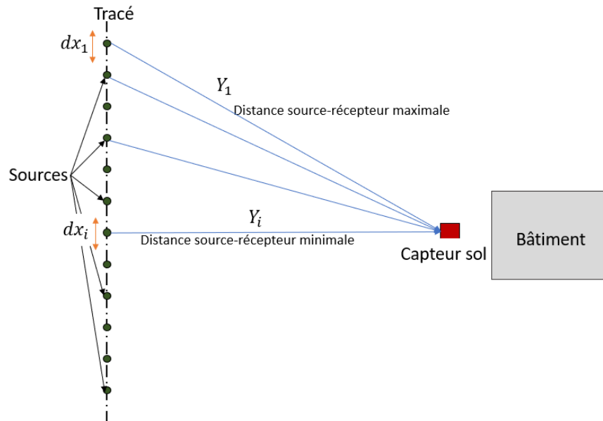
Figure 21 : Représentation de la source linéique et des mobilités de transfert ponctuelles associées (vue en plan)
