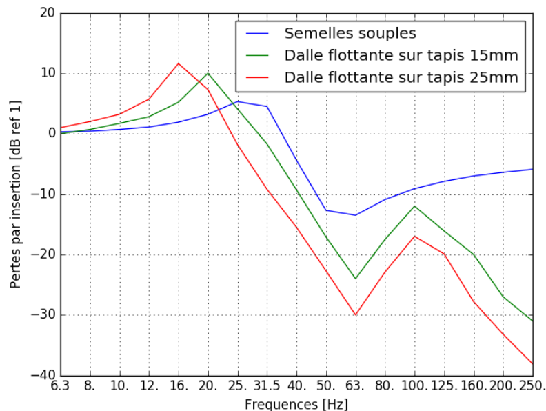
Figure 31 : Pertes par insertion calculées pour trois types de pose de voie couramment utilisés pour du tramway.
