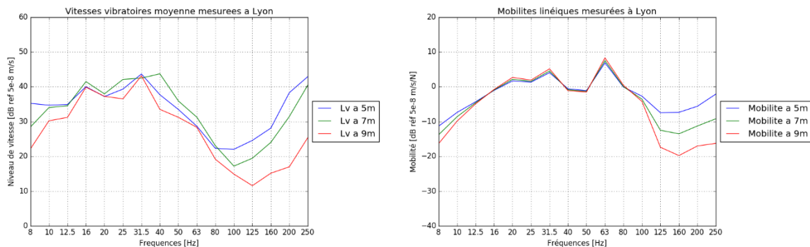
Figure 17 : Résultats intermédiaires de la campagne de mesure de niveau d'excitation Gauche : vitesses moyennes relevées aux passages des rames Droite : mobilités linéiques calculées à l'aide des mobilités ponctuelles mesurées sur site
