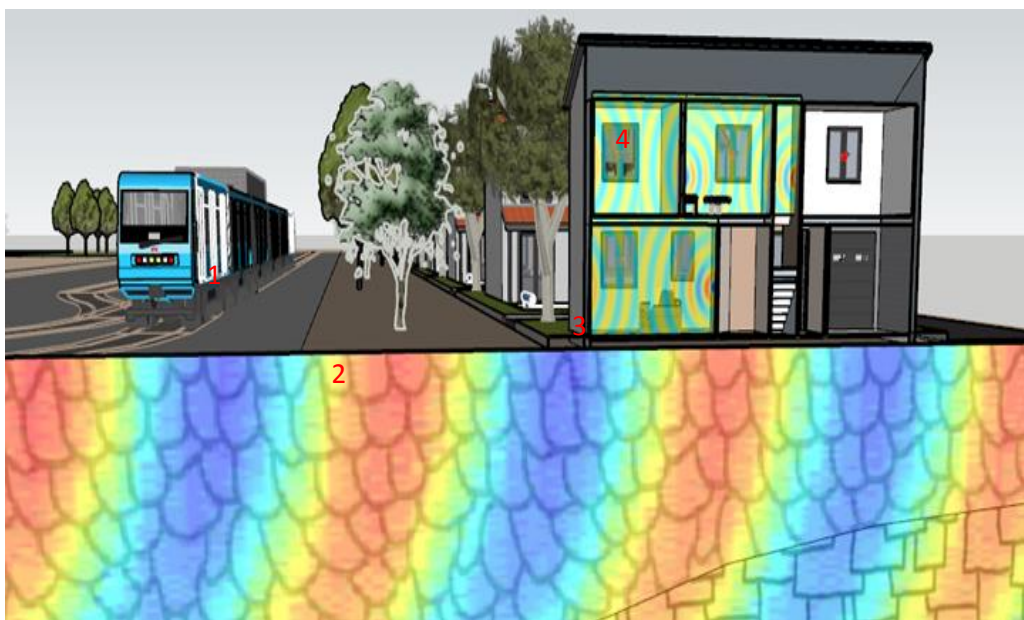
Schéma de principe de propagation des vibrations ferroviaires dans l'environnement
