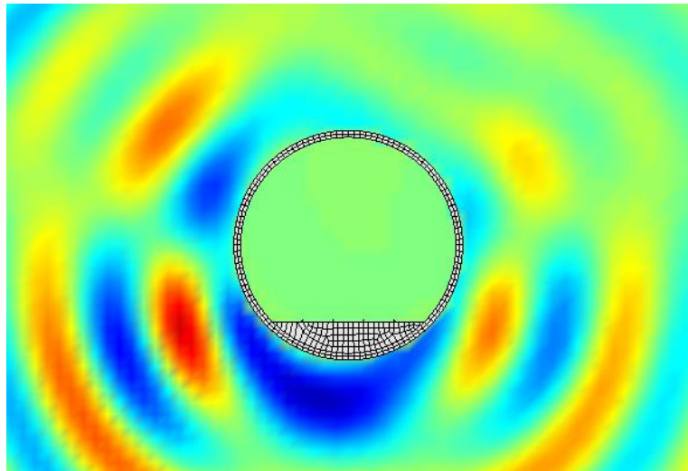
Figure 33 : Exemple de résultat de modélisation 2D½ (FEM-BEM) avec le logiciel TRAFFIC développé par KU Leuven (Champ de déplacement dans un sol excité par une force sur le radier du tunnel)
