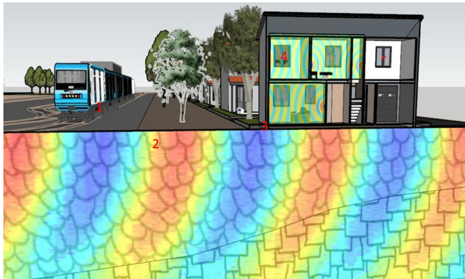
Figure 5 : Transmission des vibrations et bruits solidiens d'origine ferroviaire Cas d'un système de transport en surface (Illustration SYSTRA)
