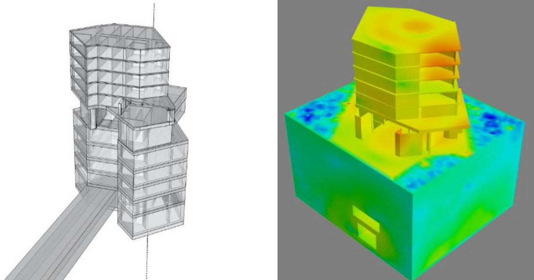
Figure 34 : Étapes d'une modélisation numérique approfondie (gauche : CAO - Droite : résultats de simulation)
