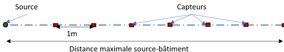
Figure 22 : Configuration des essais de décroissance dans le sol
