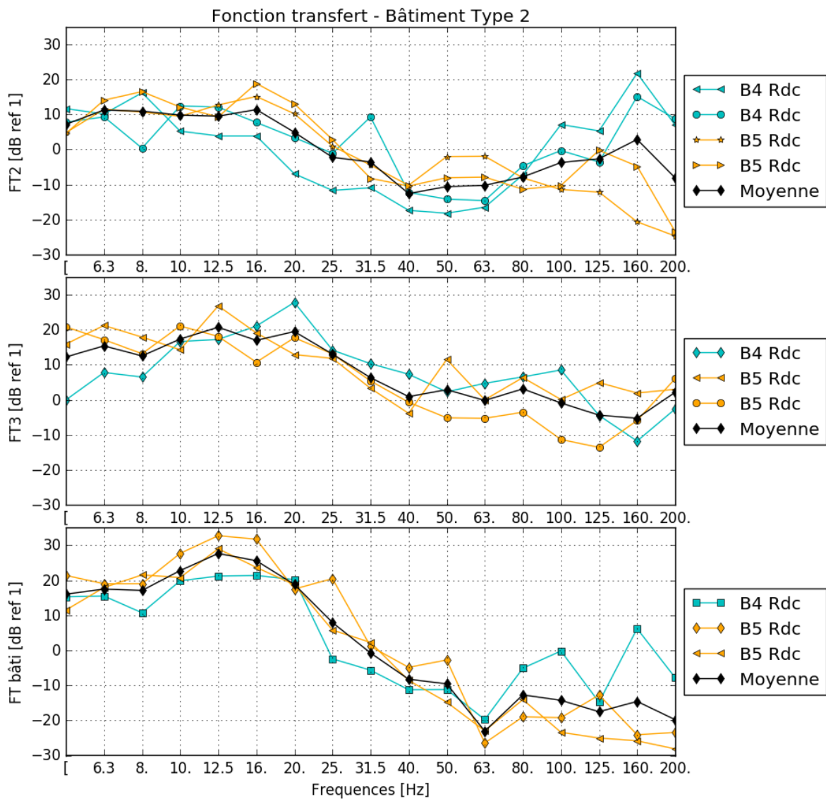
Figure 29 - Fonctions de transfert sol/bâtiment (FT2, FT3 et FTb) mesurées pour plusieurs bâtiments de type 2
