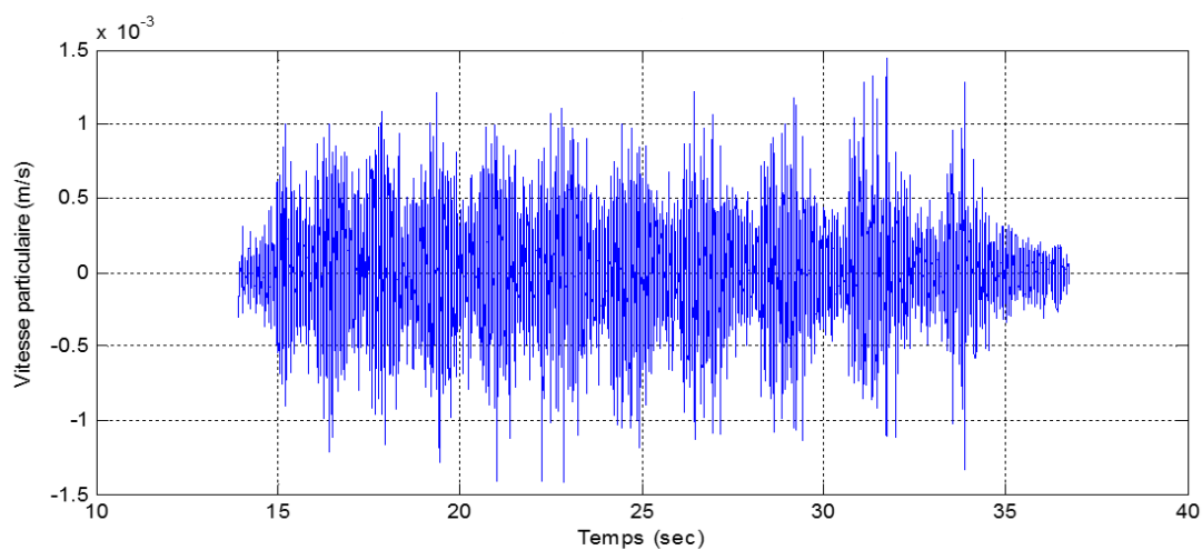
Figure 4 : Exemple de signal de vitesse vibratoire mesuré sur la plateforme en béton d'une voie ferrée d'un système de transport urbain (Illustration SYSTRA)
