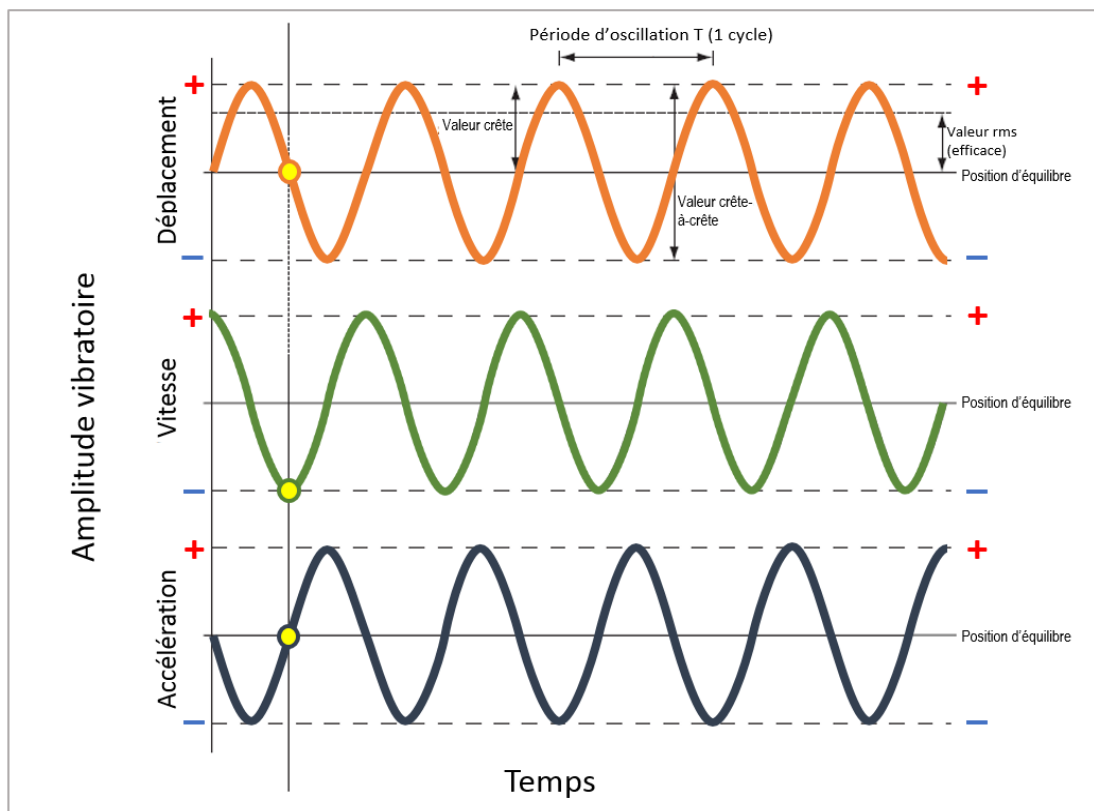
Figure 2 : Quantités utilisées pour caractériser un mouvement vibratoire
