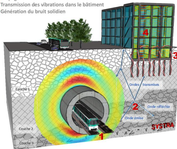
Figure 6 : Transmission des vibrations et bruits solidiens d'origine ferroviaire Cas d'un système de transport en tunnel (Illustration SYSTRA)
