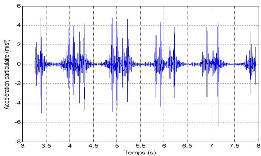
Figure 3 : Exemple de signal d'accélération vibratoire mesuré sur une traverse de la voie ferrée d'un système de transport urbain (Illustration SYSTRA)
