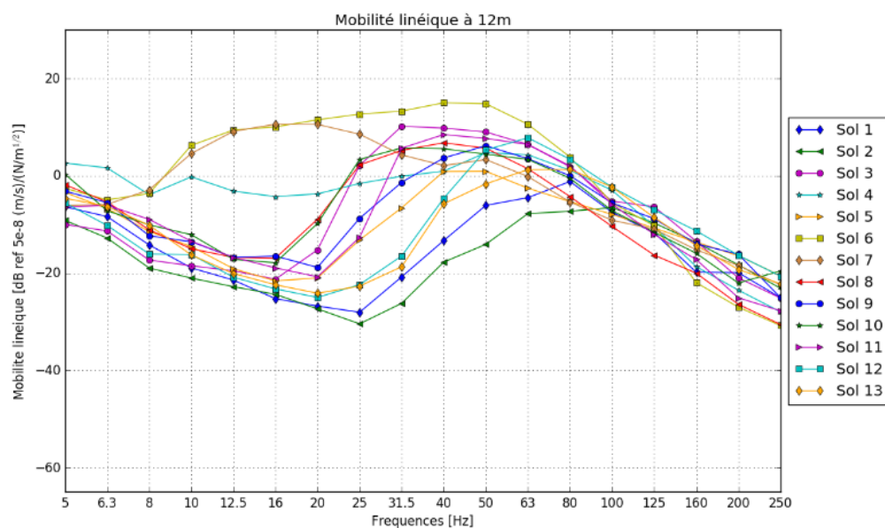
Figure 25 : Mobilités linéiques FT1 calculées à 12 m (bas)
