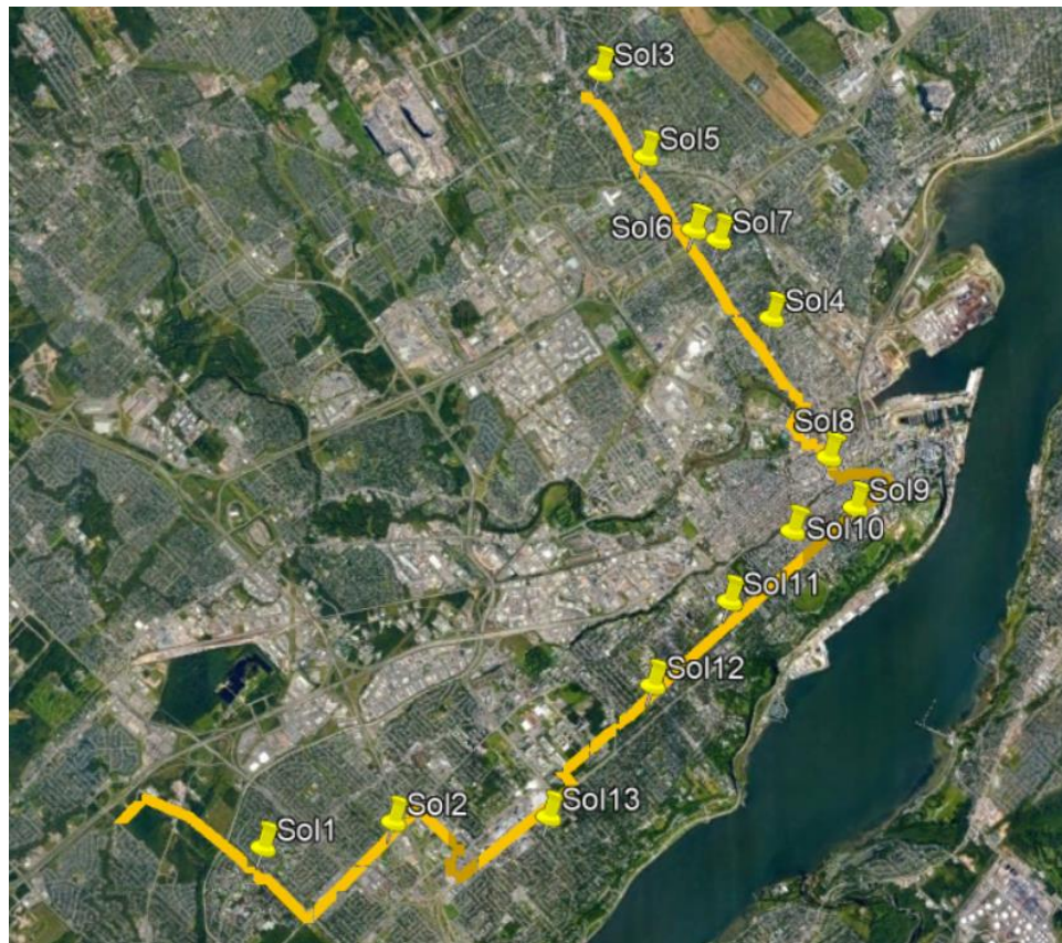
Figure 24 : Position des emplacements de mesure de décroissance dans le sol effectuée lors de la campagne d'essais (juillet 2019)
