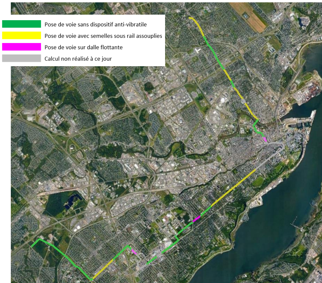
Figure 32 : Linéaire de pose de voie anti vibratile nécessaire à l'évitement de risque d'impact vibratoire (voie en surface)
