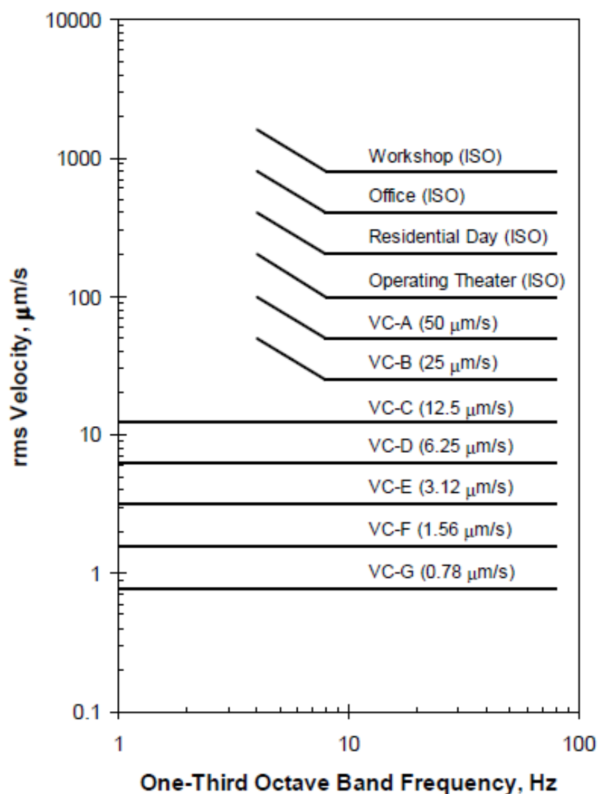
Figure 7 : Courbes génériques VC (Vibration Criterion) préconisées pour les équipements sensibles
