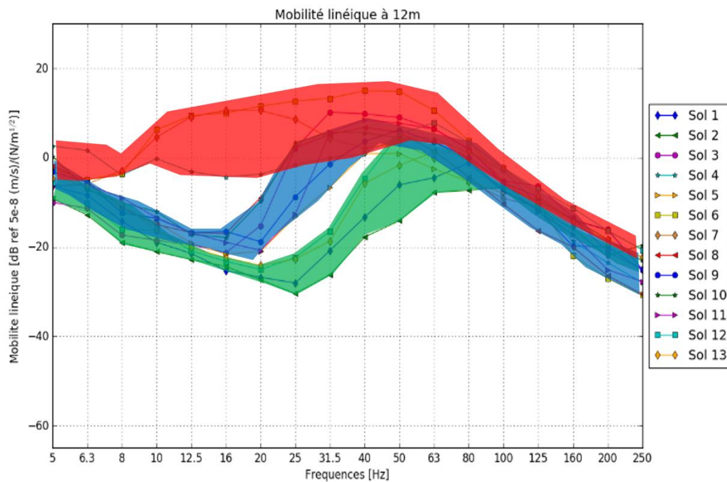
Figure 26 : Variabilité des mobilités de transfert linéiques selon le secteur considéré
