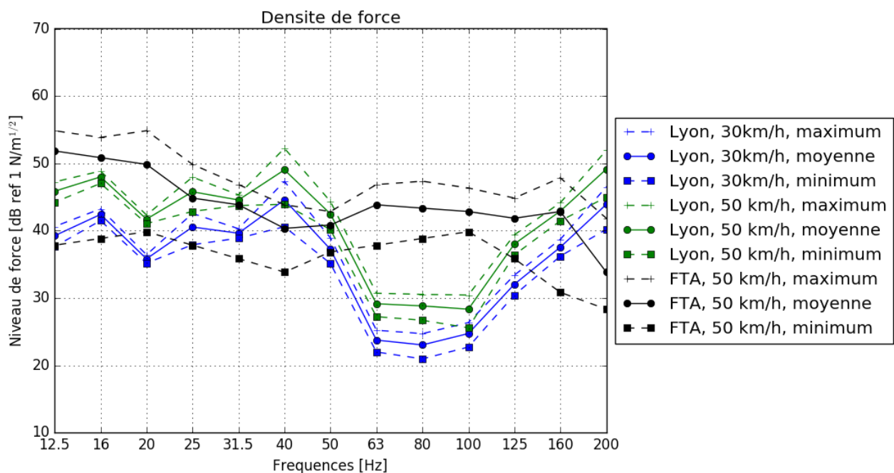
Figure 19 : Spectre densité de force appliqué sur le radier de voie pour une rame selon [1]
