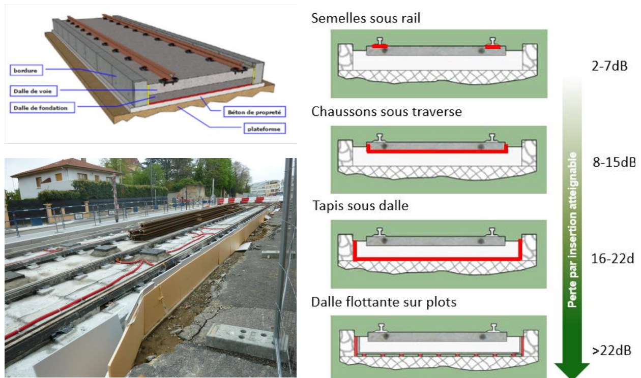
Figure 30 : Schéma de principe des moyens de mitigation usuels (dalle flottante à gauche et échelle de performance à droite) Bas gauche : réservation prévue pour une dalle flottante lors de la phase de construction
