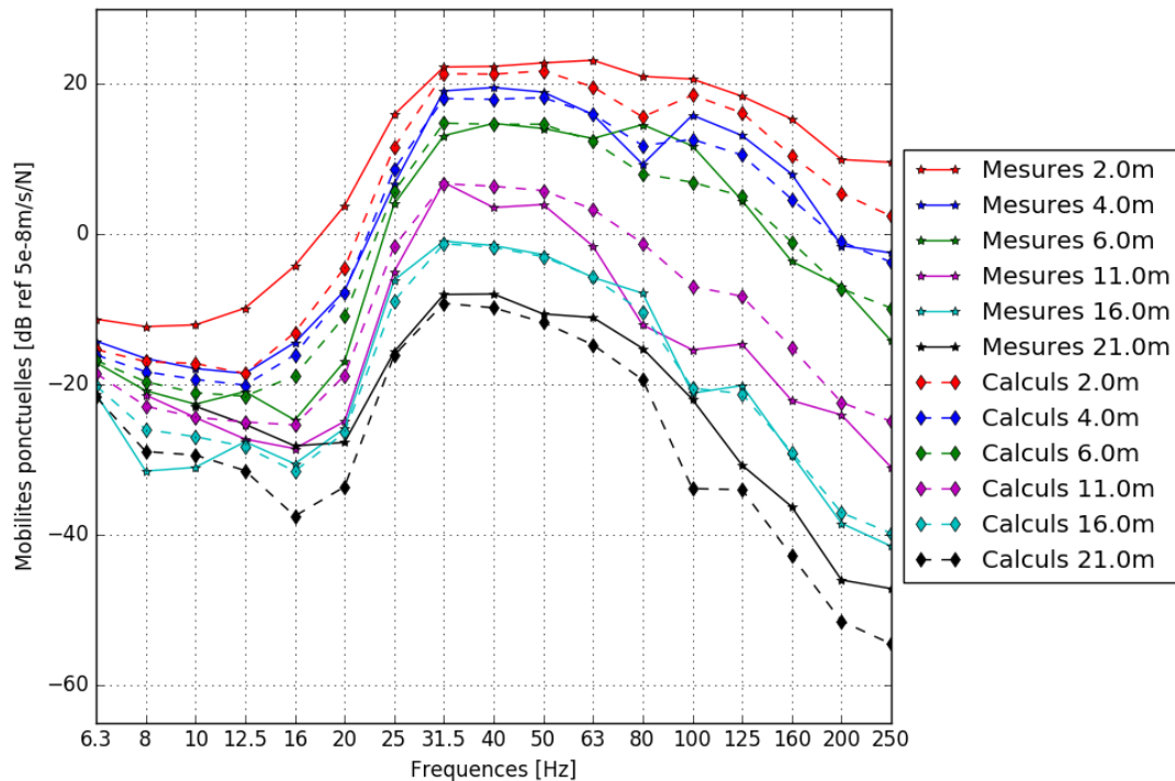
Figure 23 : Exemple de décroissance dans le sol calculée à partir des essais effectués sur le site 3
