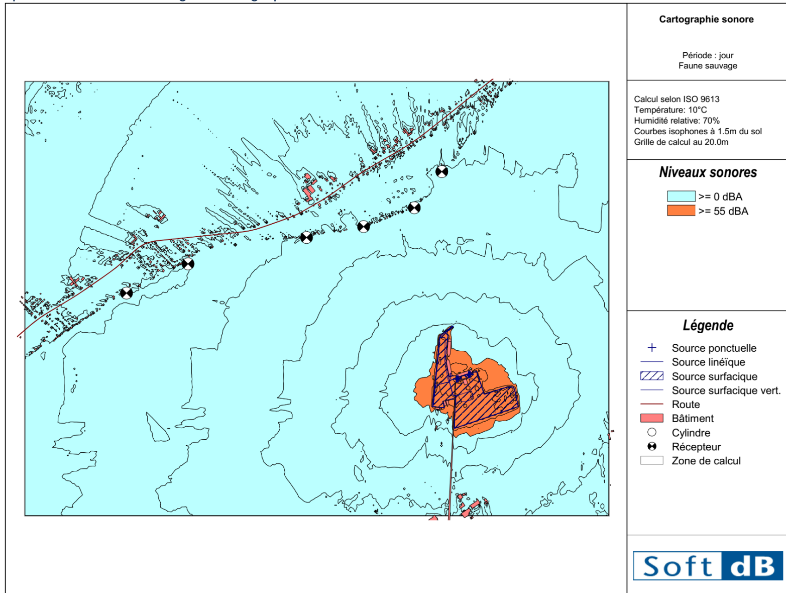
Figure 12 : Cartographie sonore L Aeq,1h à 1,5m du sol du terminal portuaire de jour – état actuel - faune sauvage (>=55 dBA)
