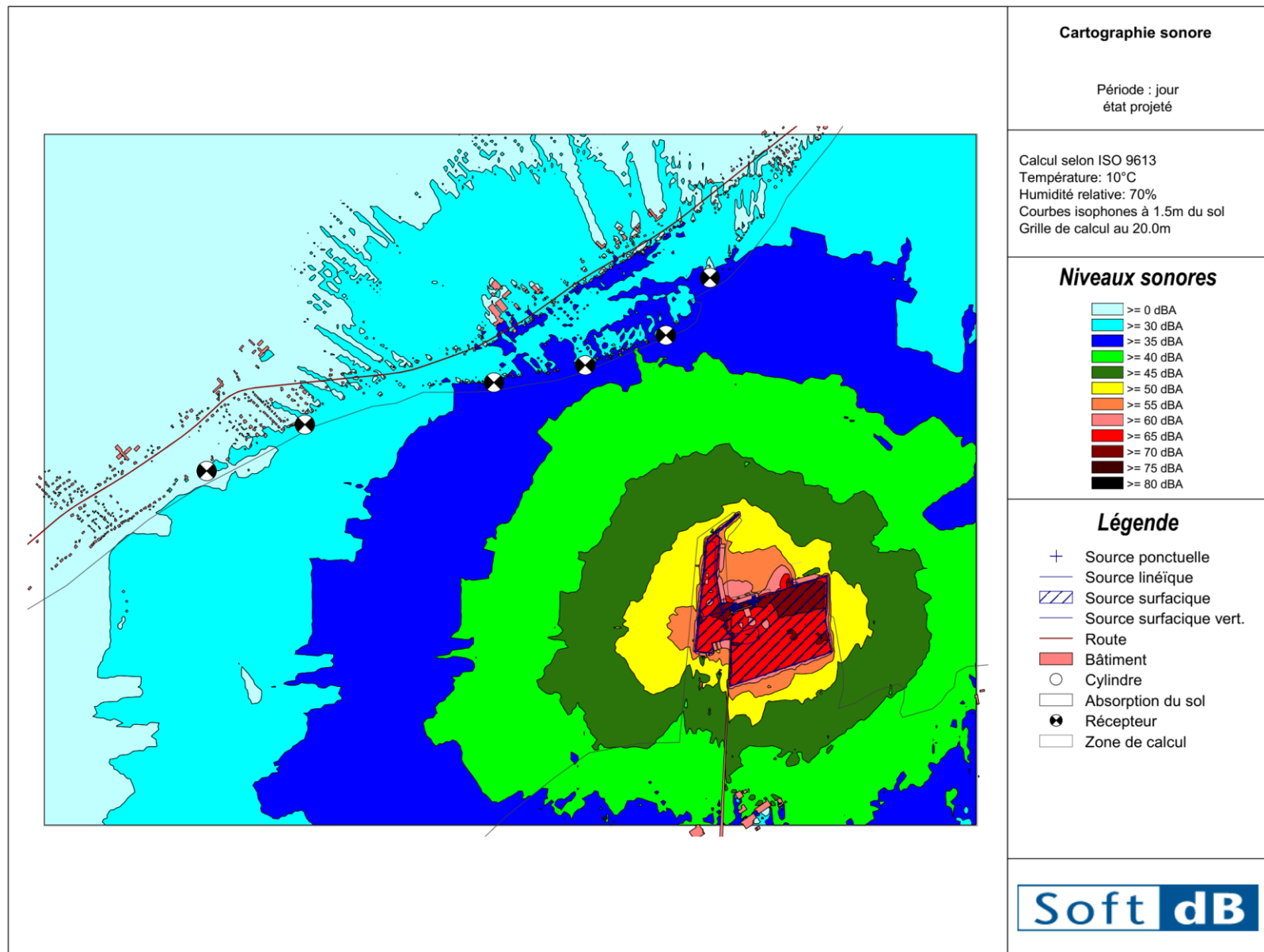
Figure 15 : Cartographie sonore LAeq,1h à 1,5m du sol du terminal portuaire de jour – état projeté
