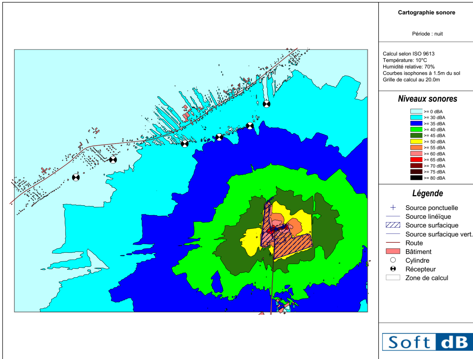
Figure 11 : Cartographie sonore L Aeq,1h à 1,5m du sol du terminal portuaire de nuit - état actuel
