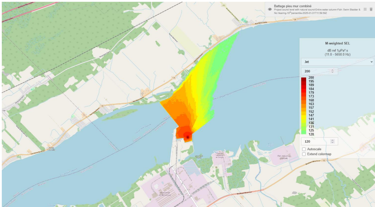
Figure 3-7 Patron de propagation du bruit généré par le battage d'un pieu de 1219 mm au mur combiné en janvier. Pression sonore à la source : 204 dB re 1 uPa @ 1 m 10 .
