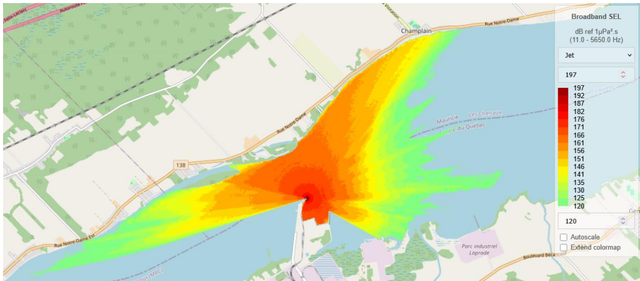
Figure 3-3 Patron de propagation du bruit généré par le vibrofonçage d'un pieu de 2286 mm au duc-d'Albe en février. Pression sonore à la source : 211 dB re 1 \mu Pa @ 1 m 6 .
