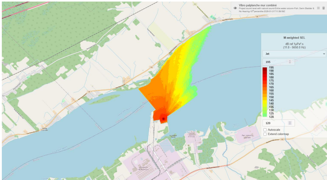
Figure 3-5 Patron de propagation du bruit généré par le vibrofonçage d'une palplanche de 1400 mm au mur combiné en janvier. Pression sonore à la source : 199 dB re 1 uPa @ 1 m 8 .
