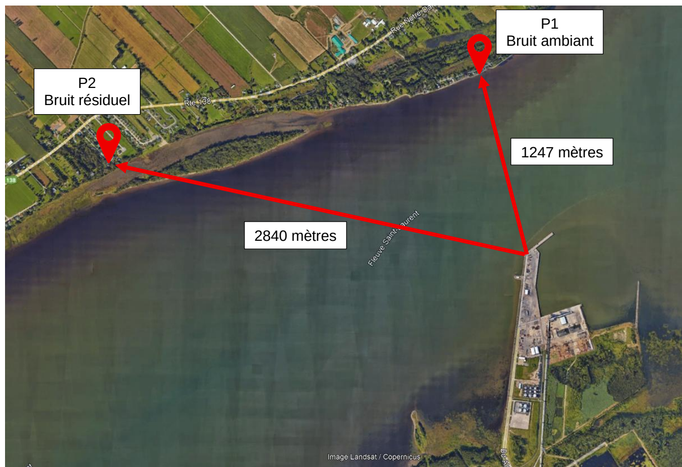
Figure 4 : Localisation des points de mesures sur le secteur d'étude
