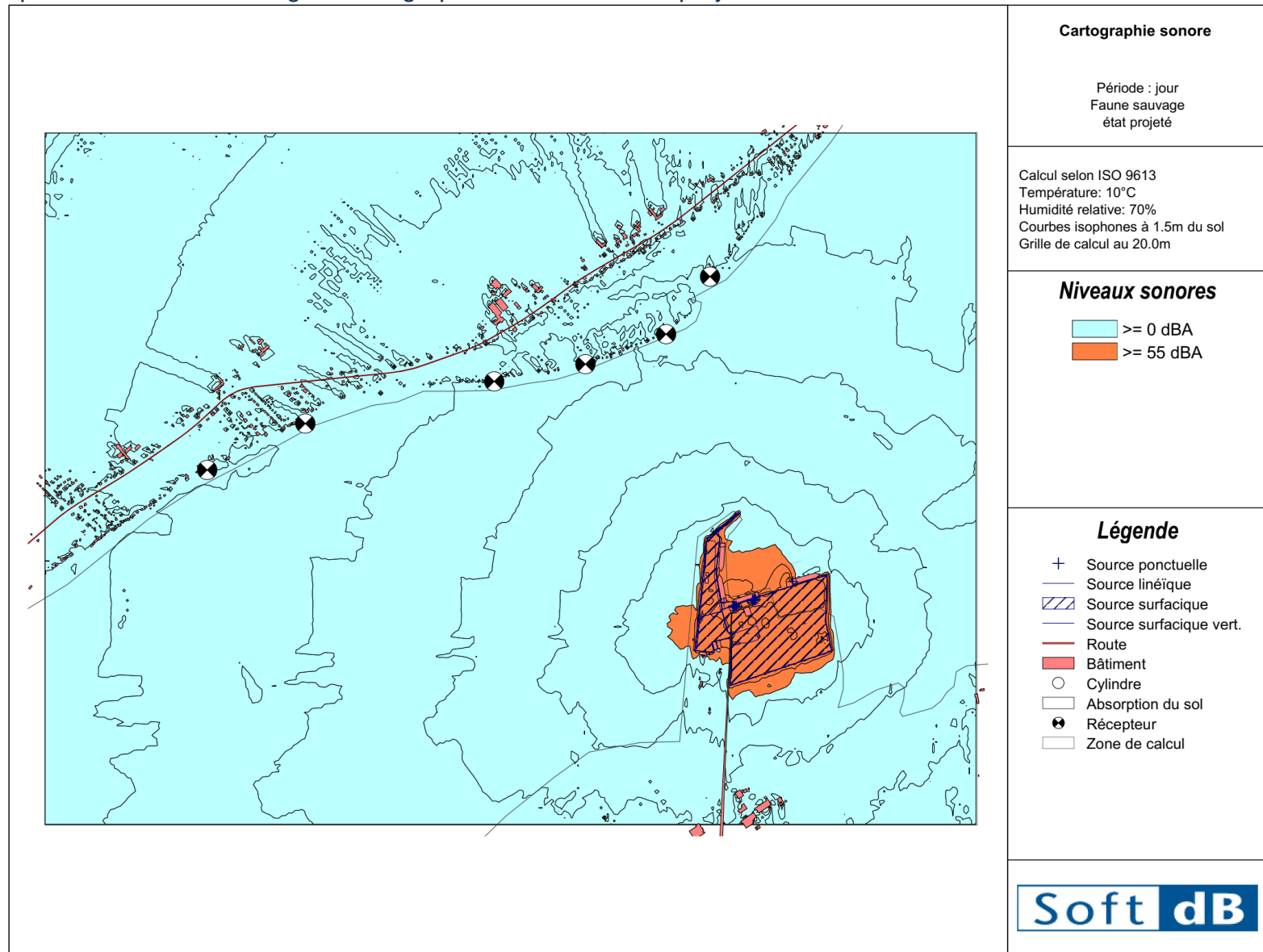
Figure 17 : Cartographie sonore L Aeq,1h à 1,5m du sol du terminal portuaire de jour – état projeté - faune sauvage (>=55 dBA)
