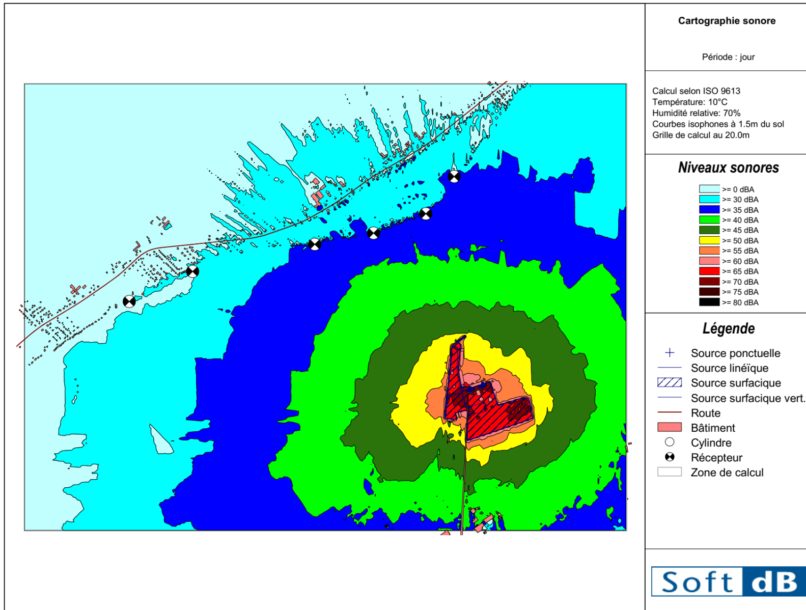
Figure 10 : Cartographie sonore LAeq,1h à 1,5m du sol du terminal portuaire de jour – état actuel
