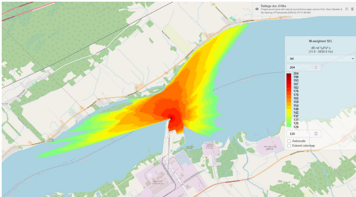
Figure 3-6 Patron de propagation du bruit généré par le battage d'un pieu de 2286 mm au duc-d'Albe en février. Pression sonore à la source : 211 dB re 1 uPa @ 1 m 9 .
