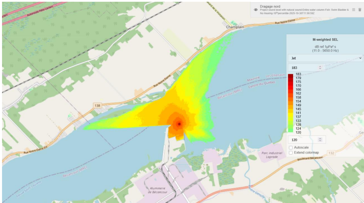
Figure 3-2 Patron de propagation du bruit généré par le forage de l'emboîture d'un pieu de 2286 mm au duc-d'Albe en avril. Pression sonore à la source : 180 dB re 1 \mu Pa @ 1 m 5 .
