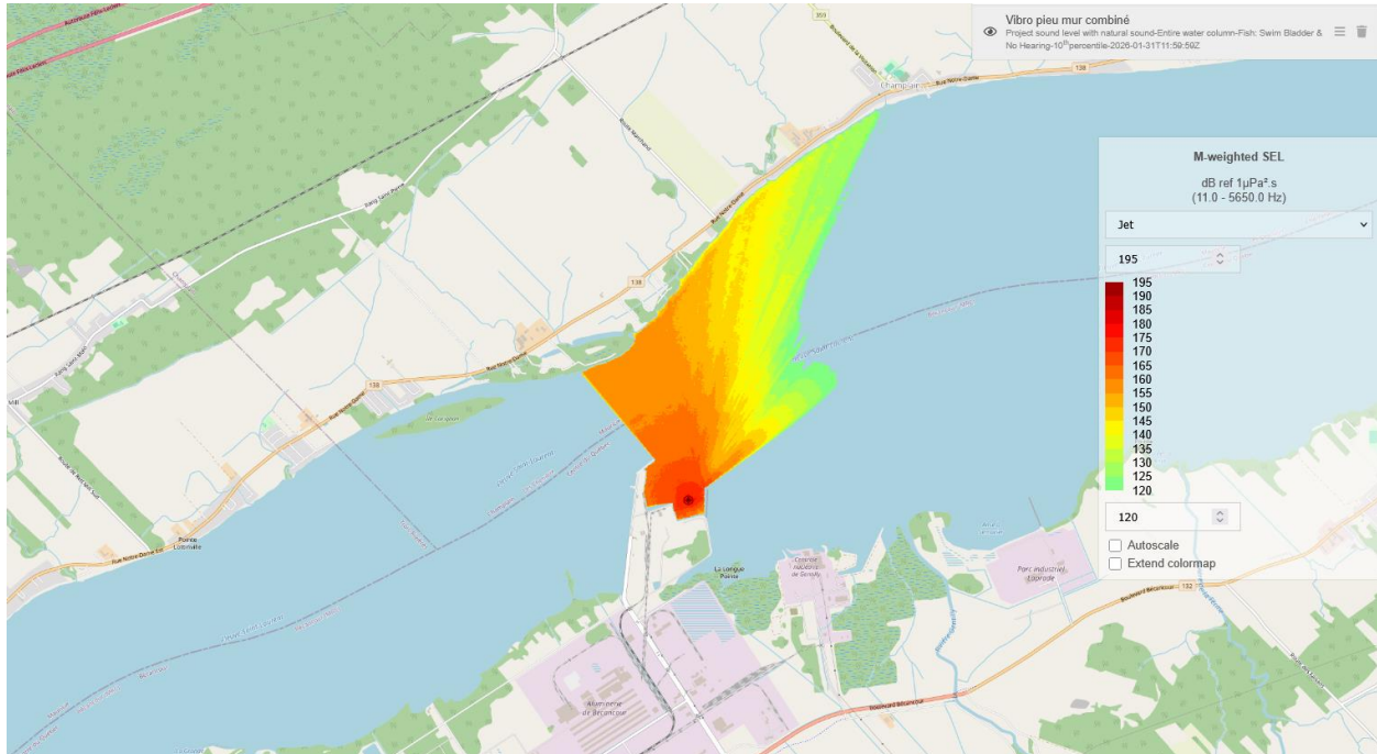
Figure 3-4 Patron de propagation du bruit généré par le vibrofonçage d'un pieu de 1219 mm au mur combiné en janvier. Pression sonore à la source : 197 dB re 1 \mu Pa @ 1 m 7 .
