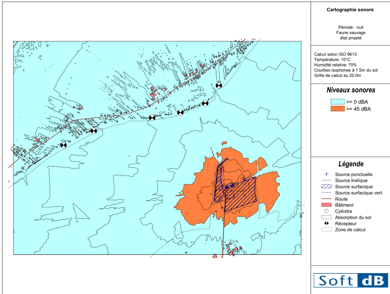
Figure 18 : Cartographie sonore LAeq,1h à 1,5m du sol du terminal portuaire de nuit - état projeté – faune sauvage (>=45 dBA)
