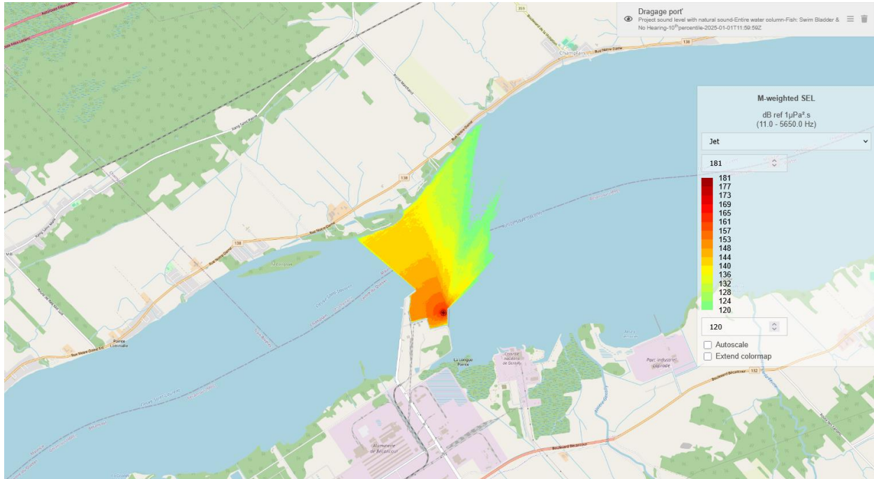
Figure 3-1 Patron de propagation du bruit de dragage à la benne preneuse à l'intérieur de la darse en janvier. Pression sonore à la source : 187 dB re 1 uPa @ 1 m 4 .
