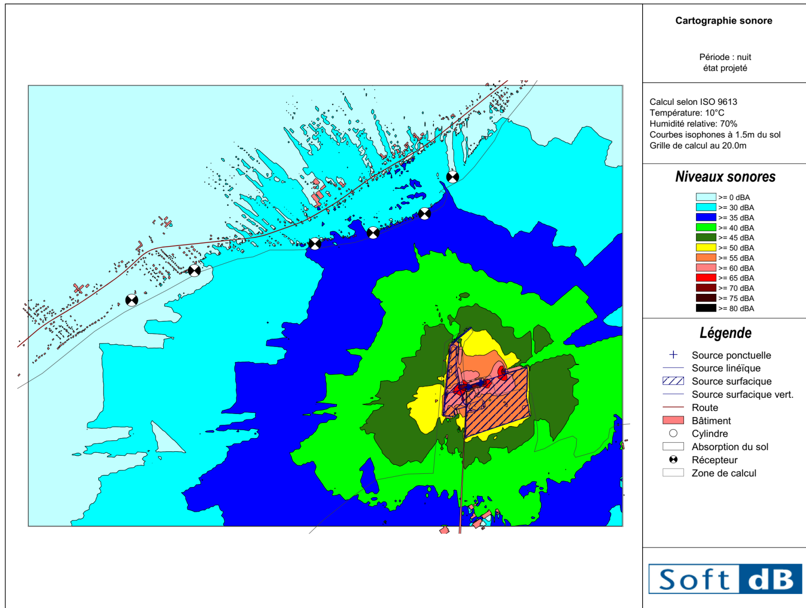
Figure 16 : Cartographie sonore LAeq,1h à 1,5m du sol du terminal portuaire de nuit - état projeté
