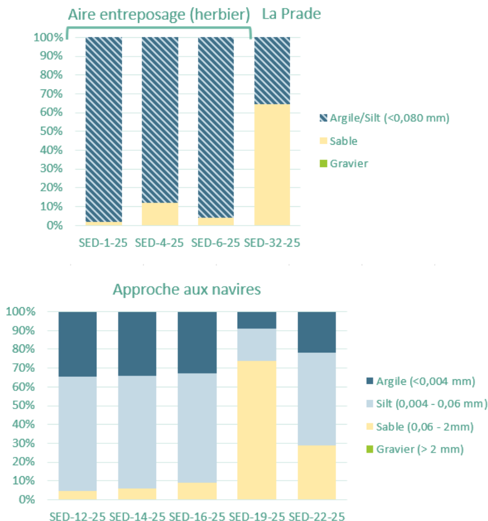
Figure 3.2 : Granulométrie et sédimentométrie des échantillons de sédiments prélevés à neuf stations (strate 0,00 à 0,30 m)
