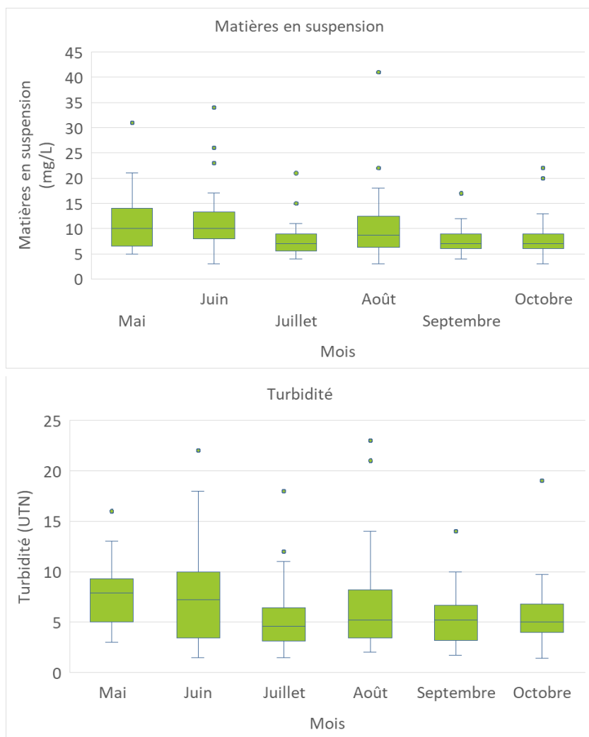
Figure 3.5 : Variabilité des concentrations de matières en suspension et des valeurs de turbidité pour les mois de mai à octobre à la station 00000092 pour les données prélevées de 1990 à 2024
