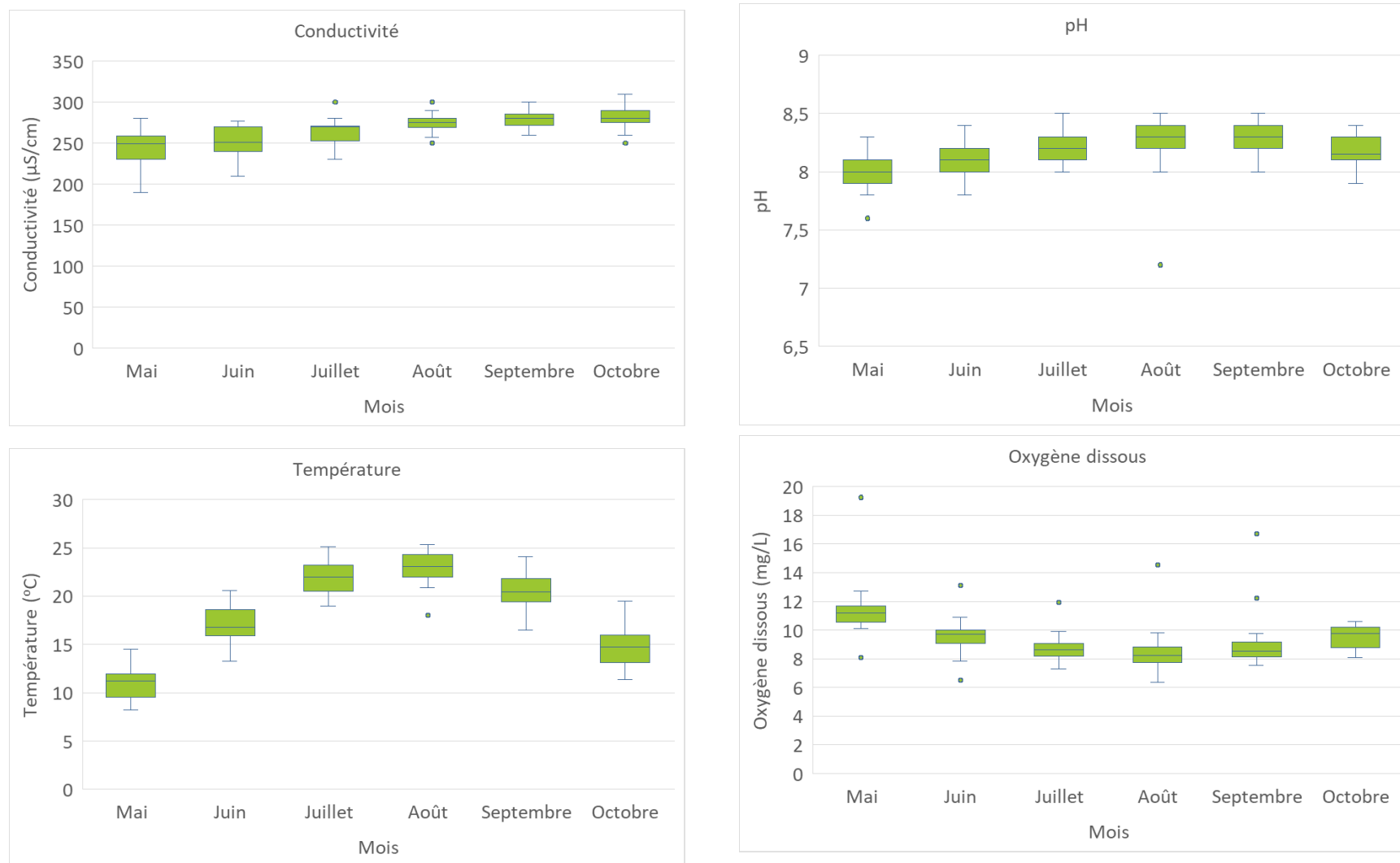
Figure 3.4 : Variabilité de la qualité de l'eau pour les mois de mai à octobre à la station 00000092 pour les données prélevées de 1990 à 2024
