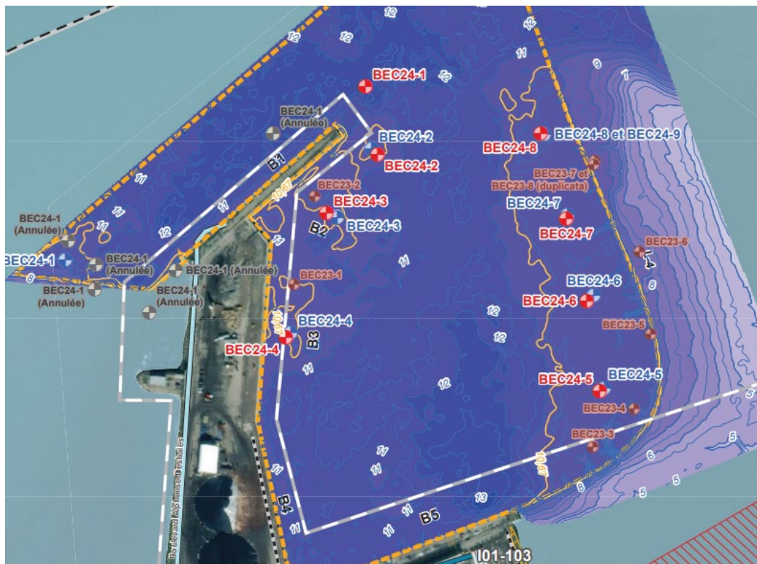
Figure 3.1 : Localisation des stations d'échantillonnage des sédiments du 20 novembre 2024
