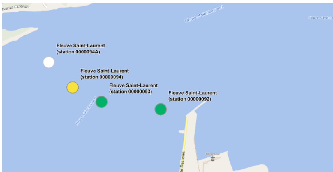
Figure 3.3 : Localisation des stations du suivi physico-chimique et bactériologique du fleuve Saint-Laurent à l’amont du port de Bécancour
