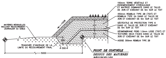
DÉTAIL TIPIQUE LIMITE D'IMPERMÉABILISATION Echelle: Aucune
