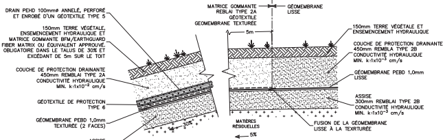
DÉTAIL TIPIQUE RECouvreMENT FINAL Echelle: Aucune
