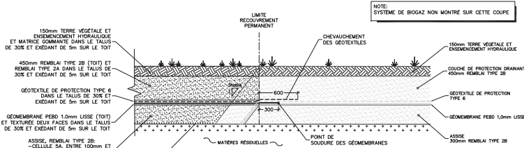
DÉTAIL TIPIQUE LIMITE DU RECouvreMENT FINAL Echelle: Aucune
