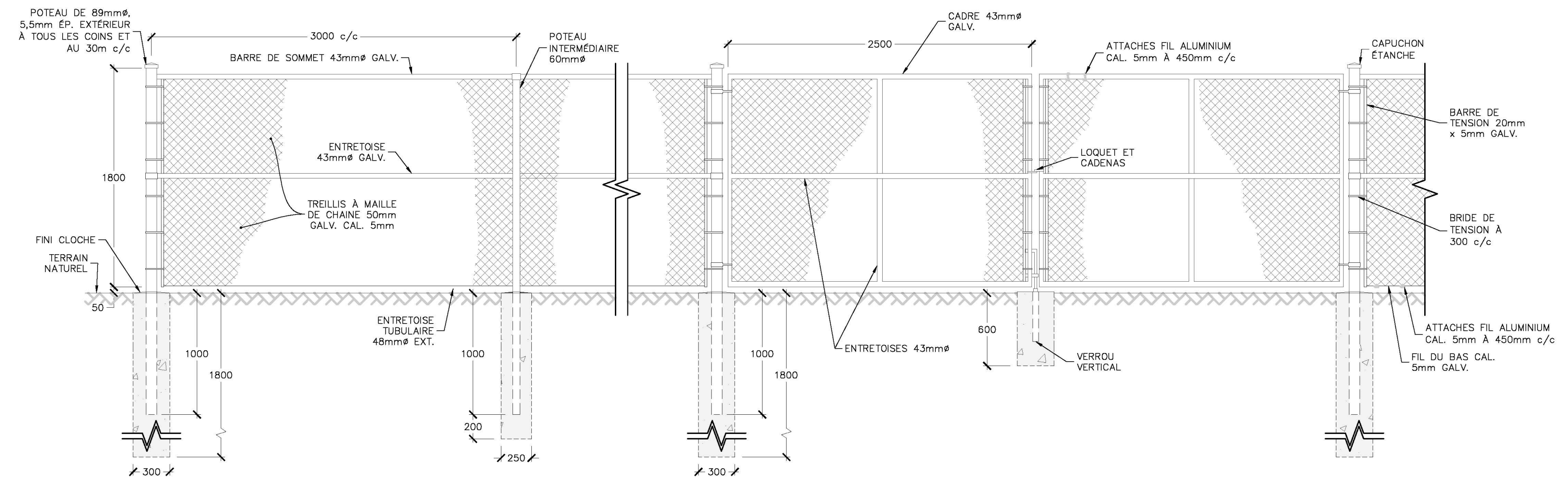
DÉTAIL TYPIQUE CLÔTURE EXISTANTE AVEC BARRIÈRE À DÉPLACER ET RÉINSTALLER ET NOUVELLE CLÔTURE ET BARRIÈRES À INSTALLER Échelle: aucune
