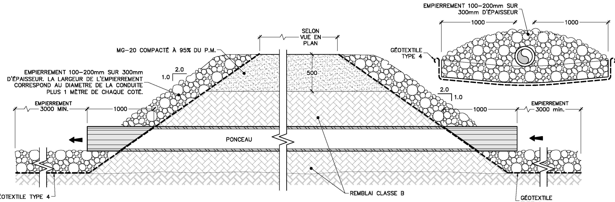
COUPE TYPIQUE PONCEAU Échelle: aucune
