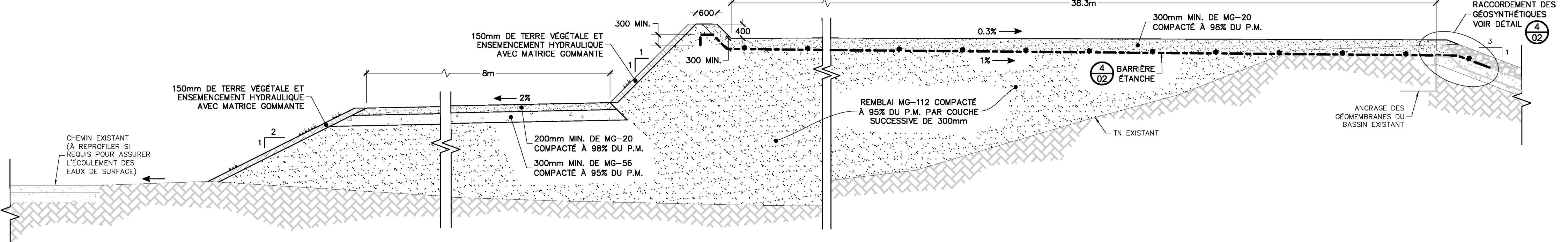
COUPE TYPIQUE PLATEFORME ÉTANCHE POUR SAC DE DÉSHYDRATATION Échelle: aucune
