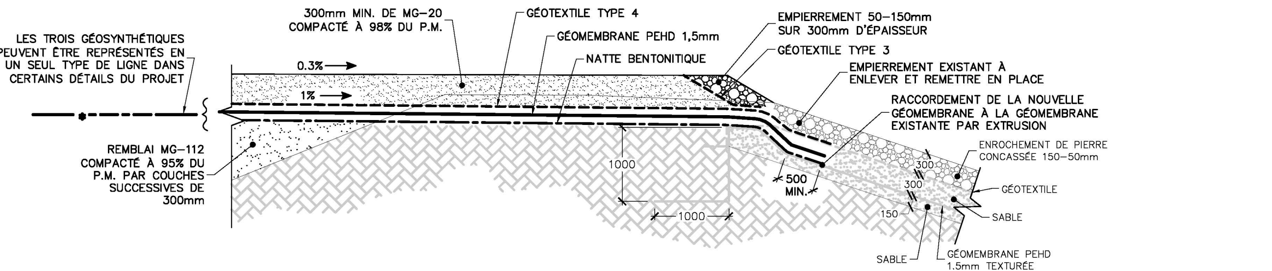
DÉTAIL TYPIQUE BARRIÈRE ÉTANCHE Échelle: Aucune
