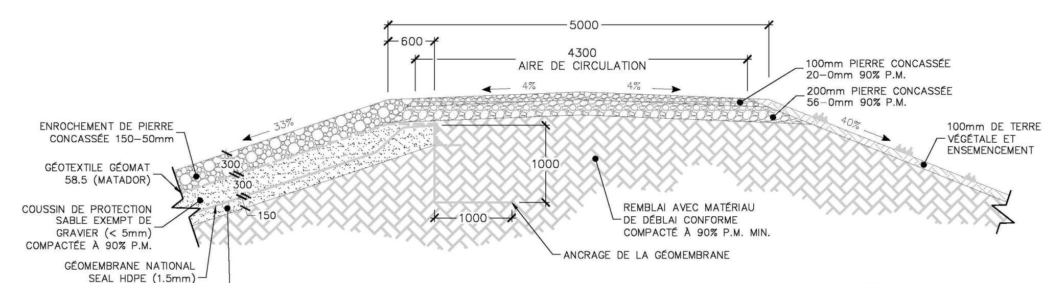
DÉTAIL TYPIQUE TRANCHÉE D'ANCRAGE DU BASSIN EXISTANT Échelle: Aucune
