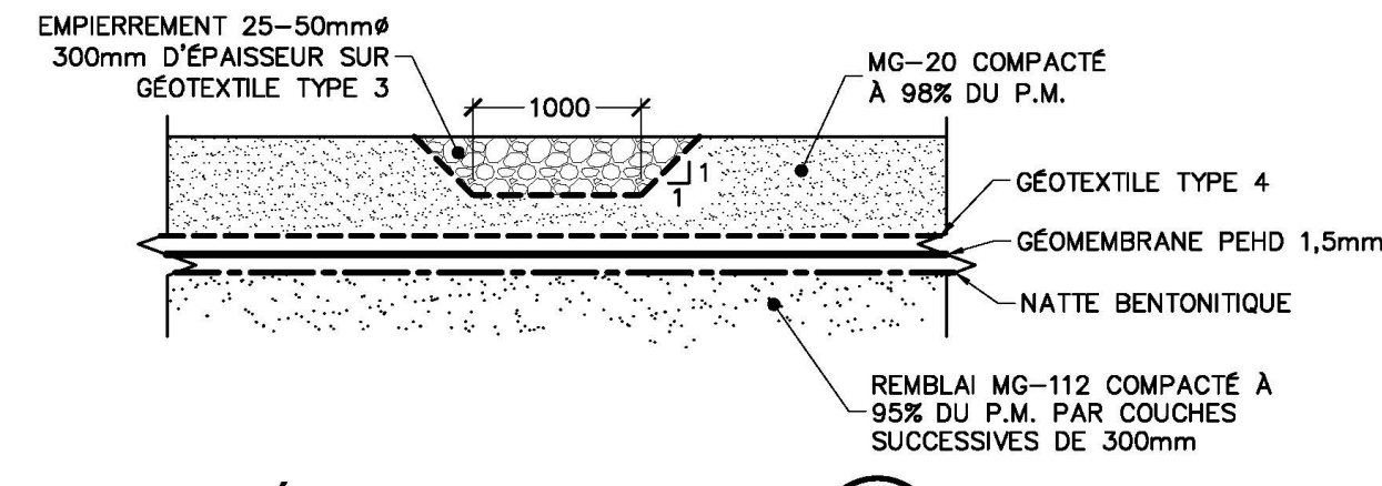
DÉTAIL TYPIQUE TRANCHÉE EMPIERRÉE Échelle: aucune
