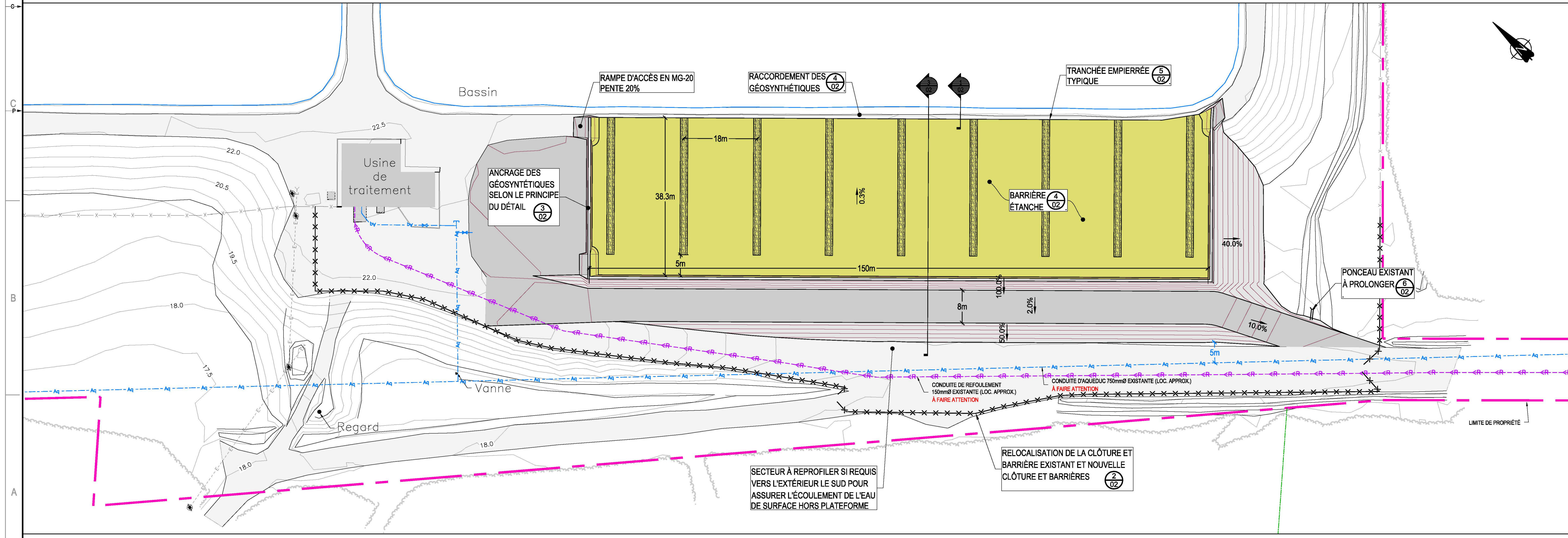
VUE EN PLAN DES TRAVAUX PROJETÉS
