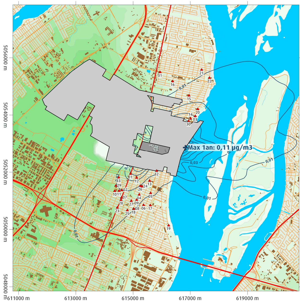
Scénario 2 (futur en mode d'opération normal) Concentrations maximales ( \mu\text{g}/\text{m}^3 ) pour le brome – Période de 1 an Pour les années 2008 à 2012
