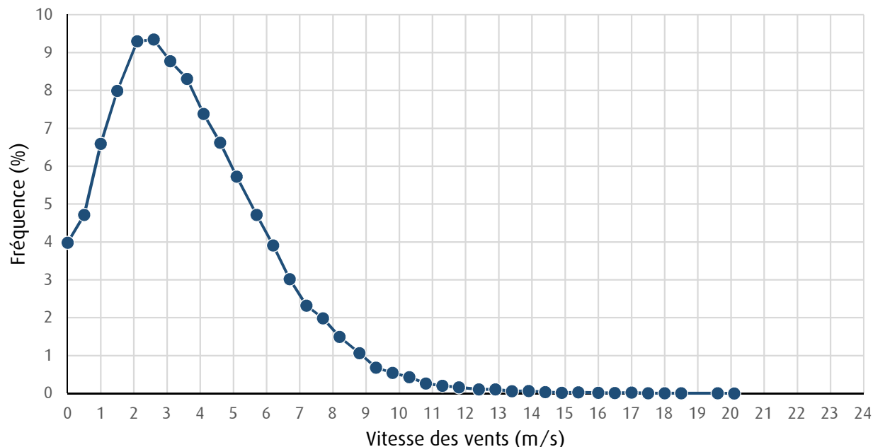
Figure 4-2 Distribution de la vitesse des vents pour la station météorologique de l'aéroport Pierre-Elliott-Trudeau de 2008 à 2012
