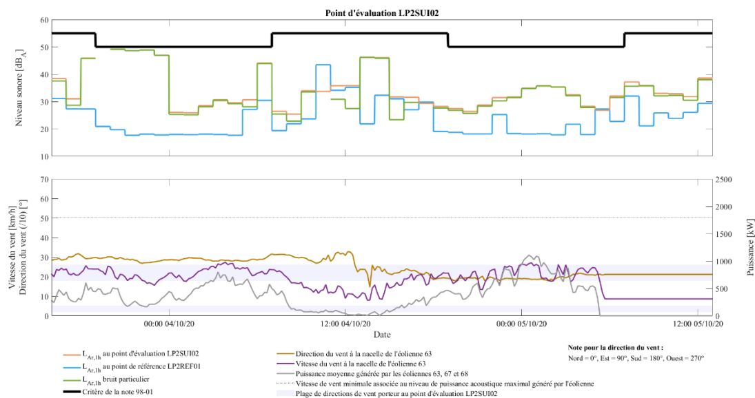
Figure 3 Niveaux sonores enregistrés au point d'évaluation LP2-SUI-02 entre le 3 et le 5 octobre 2020 – Parc éolien Le Plateau 2
