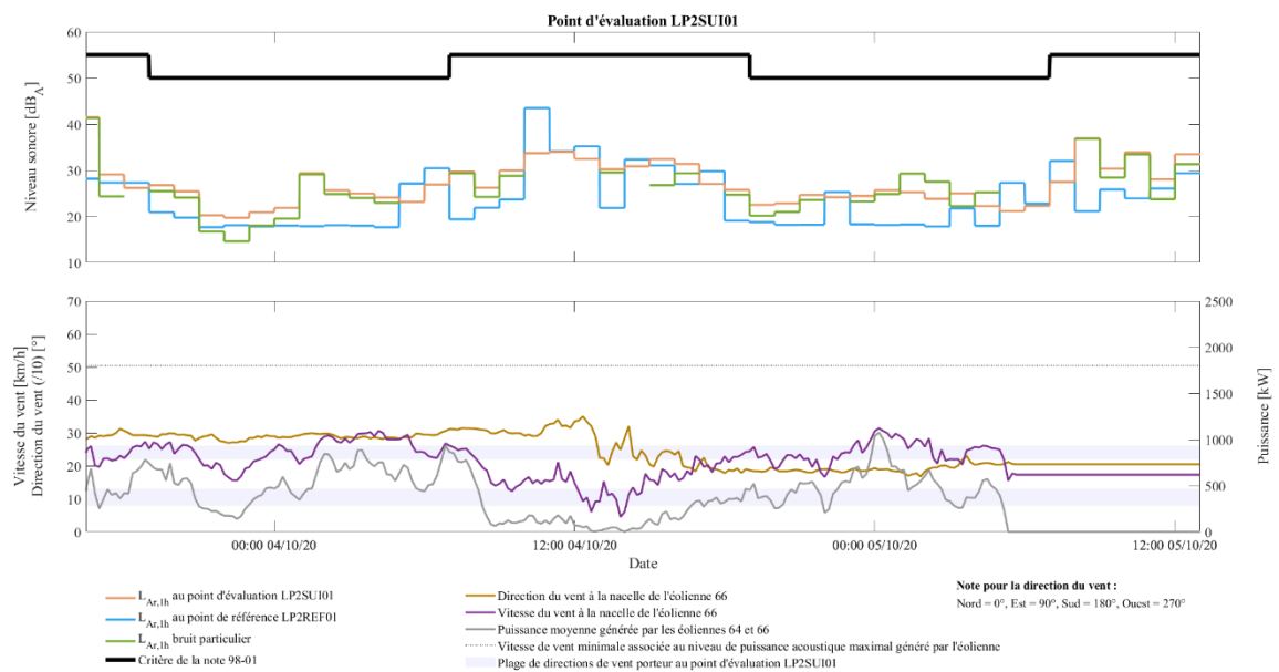
Figure 2 Niveaux sonores enregistrés au point d'évaluation LP2-SUI-01 entre le 3 et le 5 octobre 2020 – Parc éolien Le Plateau 2
